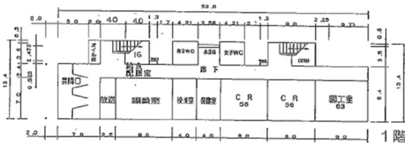
管理教室棟 ②-3R3-1864
