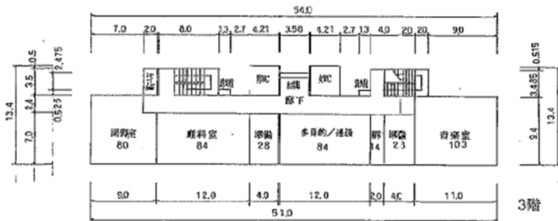
管理教室棟 ②-3R3-1864
