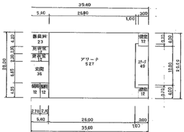
屋内運動場 ⑤-S1-708
