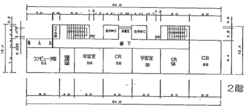
管理教室棟 ②-3R3-1864
