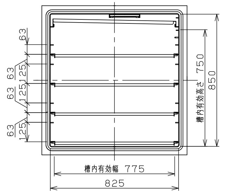
冷却槽拡大図
